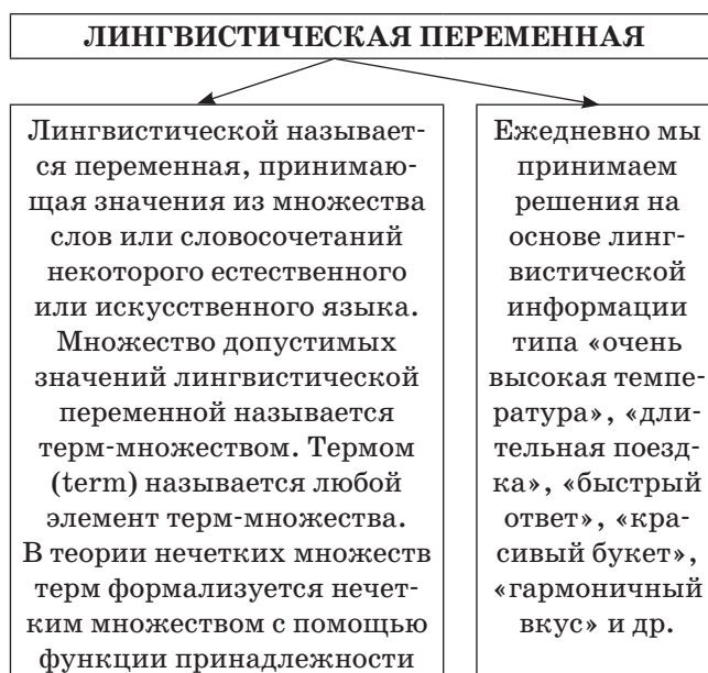
Рис. 5. К вопросу о понятии «лингвистическая переменная»
