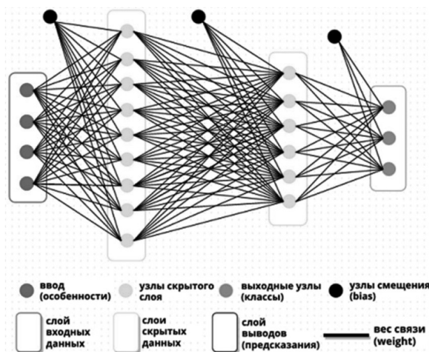
Рис. 3. Полносвязная глубокая нейросеть (коннектом)
